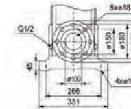
PN 16/DN 100
