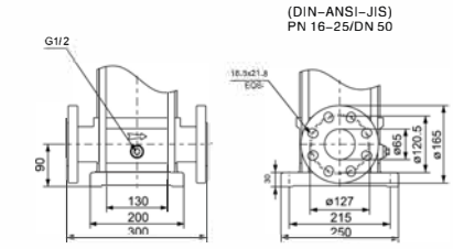
DIN FLANGE(TVS)/F
