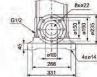
PN 25-40/DN 100
