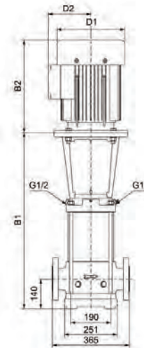
DIN FLANGE(TVS)/F
