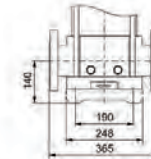
DIN FLANGE(TVR)/F
