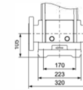
DIN FLANGE(TVR)/F
