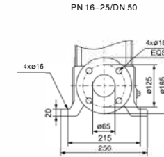
DIN FLANGE(TVR)/F
