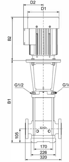
DIN FLANGE(TVS)/F
