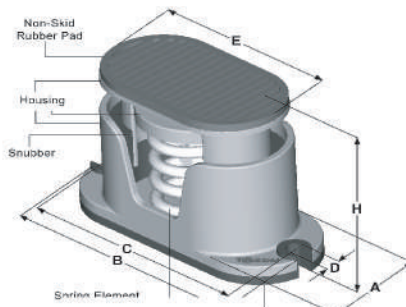
PTM-CG, PTM-CG2
