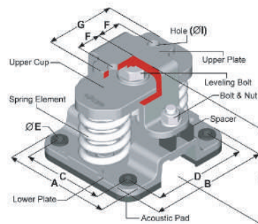
PTM-D-1652, 2202 , 2802 PTM-D2 1502, 2102
