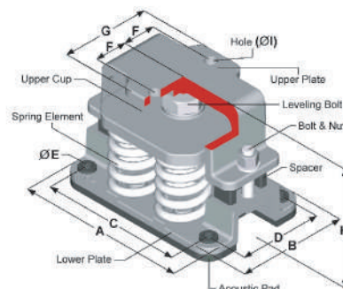
PTM-D-3304 , 4404 , 560 PTM-D2 3004, 4204
